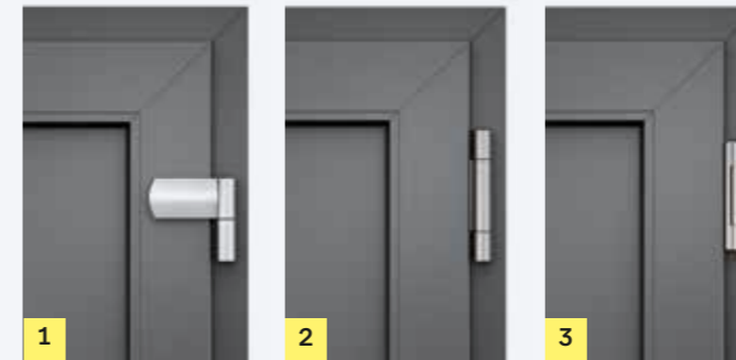
1 | Aufschraubband. (AVIDA) 2 | Rollenband. (AVIDA) 3 | Aufschraubrollenband (TERSA)
